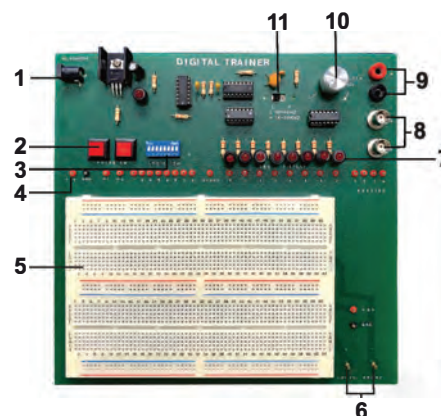
■ DT-01 Лабораторный набор для сборки цифровых цепей
