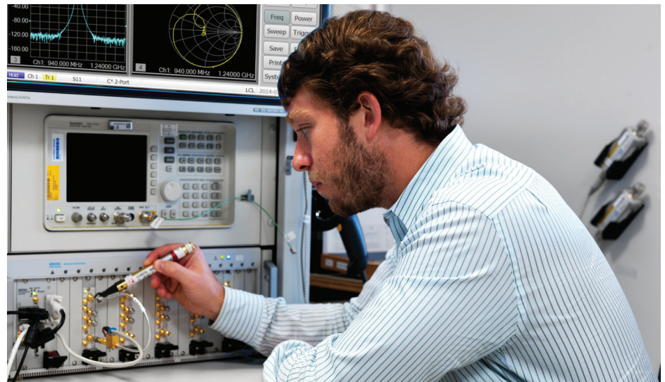
Рис. 1: Добавление к существующей испытательной установке двух 2-портовых векторных анализаторов цепей в формате PXI позволяет создать мощное средство для тестирования параметров устройств, не увеличивая при этом высоту системы тестирования или занимаемую ею площадь.
