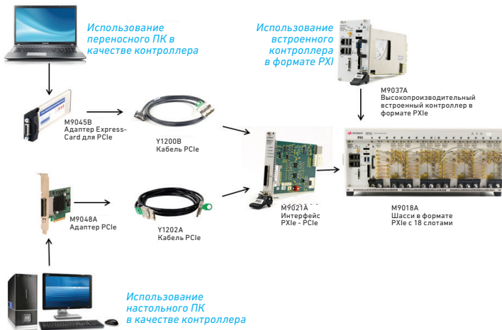
Общий обзор шасси, компьютеров, контроллеров и кабельных соединений
