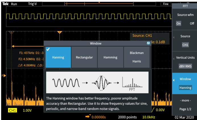
Рисунок 7. Подсказки HelpEverywhere® объясняют важные настройки.
