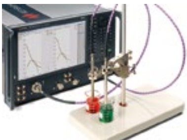
Система миллиметрового диапазона N5290A/91A с одним циклом свипирования 500 Гц до 110/120 ГГц
