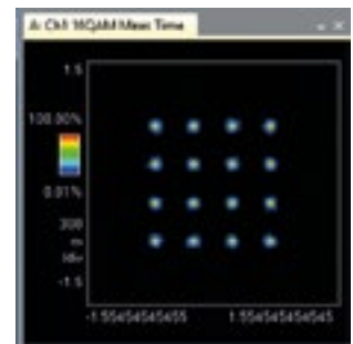
Сигнал QAM16, генерируемый на скорости 64 Гбод
