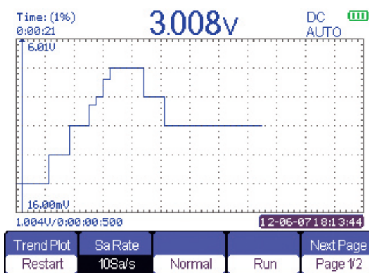
Экран регистратора (TREND PLOT в режиме Мультиметр)
