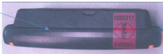
Рисунок 2 – Схема пломбировки измерительного прибора Testo 420 с датчиками с нанесением знака поверки
